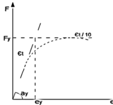
Gambar 8.1 Standar pengujian berdasarkan ECCS 1986
