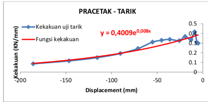
Gambar 9.3 Kekakuan fungsi displacement tarik STRS
