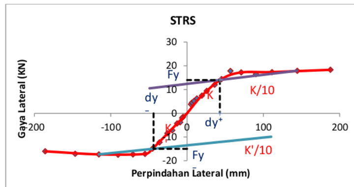
Gambar 8.3 Beban leleh dan displacemen leleh sambungan pracetak
