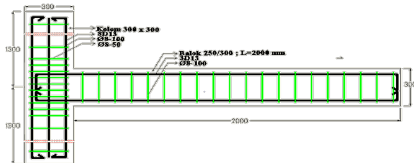
Gambar 2 Balok kolom monolit
