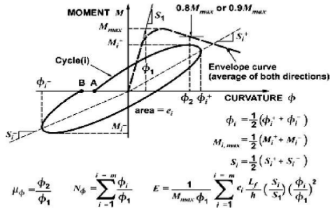
Gambar 1 Definisi dari parameter daktilitas
