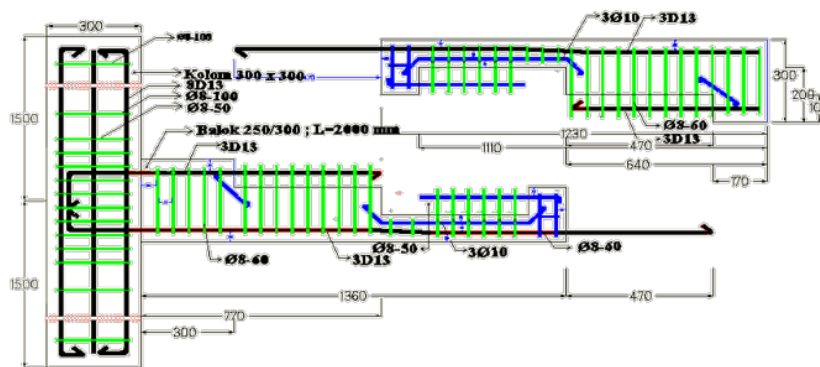
Gambar 3 Sambungan takikan lurus rangkap (STRS)
