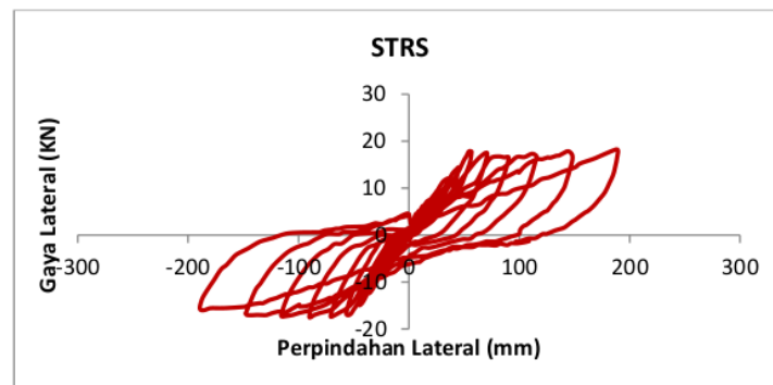
Gambar 7.2 Kurva hysteresis beban– displacement pada kolom STRS
