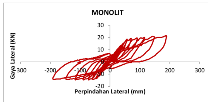
Gambar 7.1 Kurva hysteresis beban– displacement pada kolom Monolit
