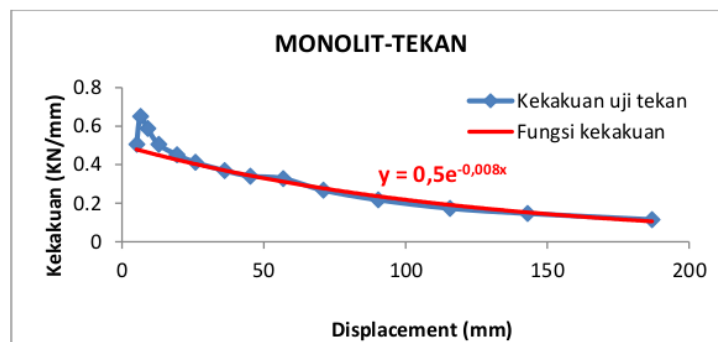
Gambar 9.2 Kekakuan fungsi displacement tarik Monolit
